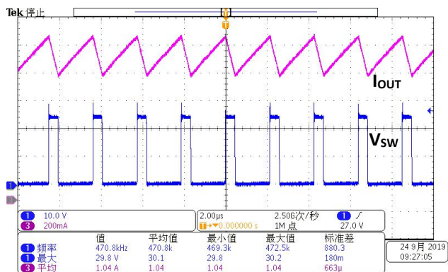
VDD=24V, VOUT=6LEDS
