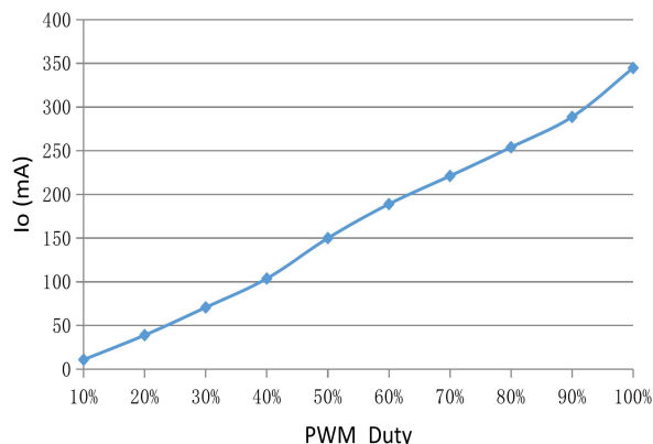
PWM特性曲线
