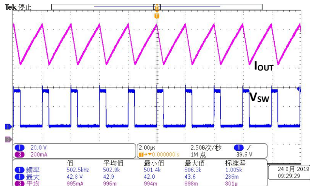
VDD=36V, VOUT=9LEDS
