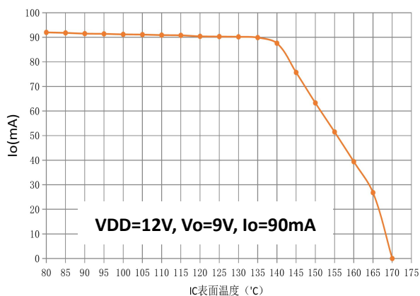
OTP特性曲线
